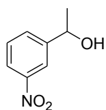
1-(3-nitrofenyl)ethanol
