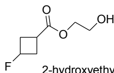
2-hydroxyethyl-3-fluorcyklobutankarboxylát
