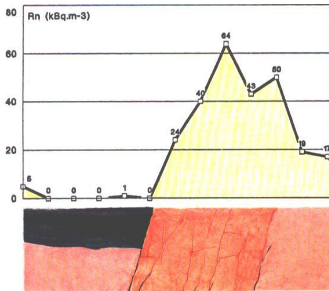
Vliv nepropustného jílovitého pokryvu na snížení hodnoty objemové aktivity radonu. Pod jílovou vrstvou vzniká bariérový efekt, radon migruje podél tektonické poruchy (lokality Radvanov u Milevska).
