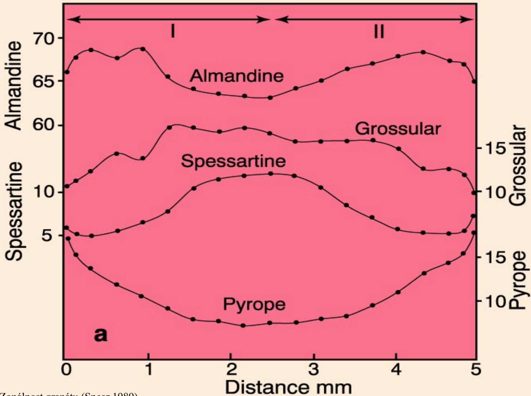
Zonálnost granátu (Spear 1989)
