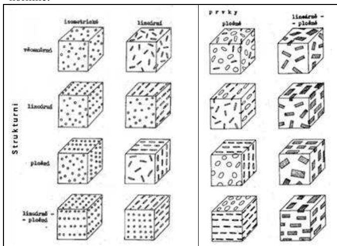
Obr. 24 Klasifikace anizotropních staveb podle Demla (1954).
