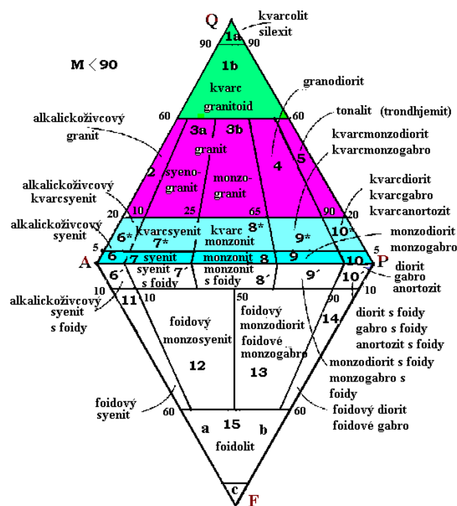
Obr. 3 QAPF_ zdvojený trojúhelníkový diagram pro plutonické horniny
