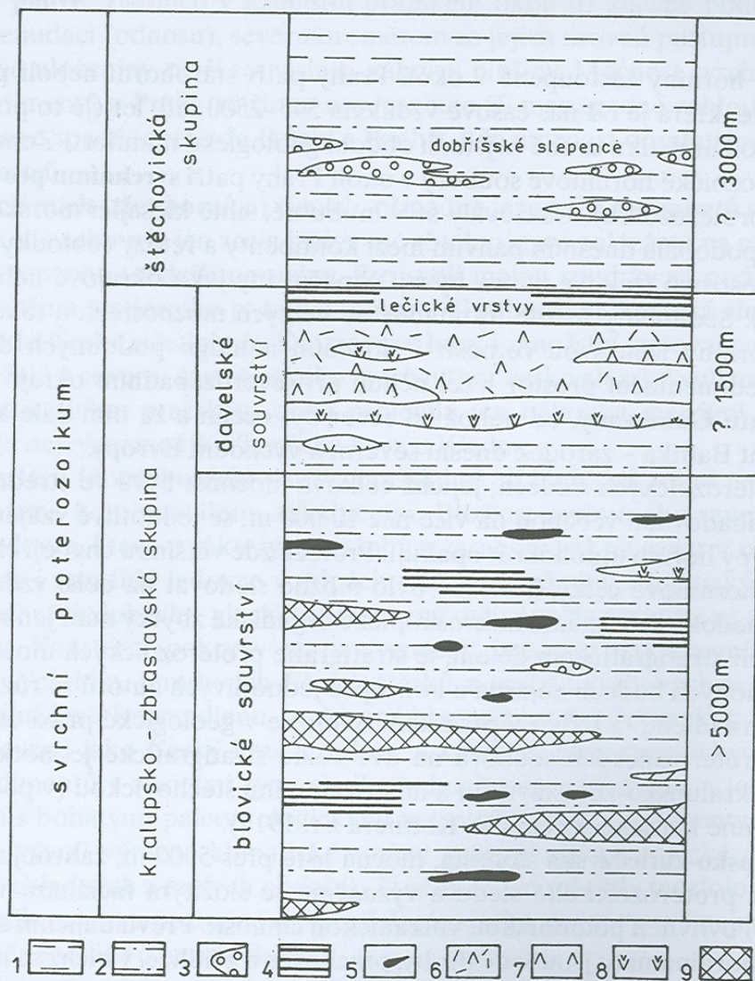
Obr. 4. Stratigrafické schéma proterozoika Barrandieny (podle J. Maška 1982).
