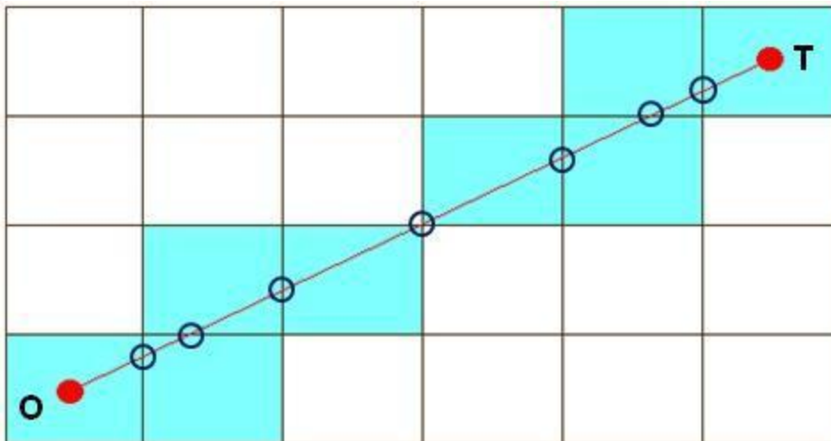
Kartografické modelování
