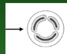
diktyostélé
