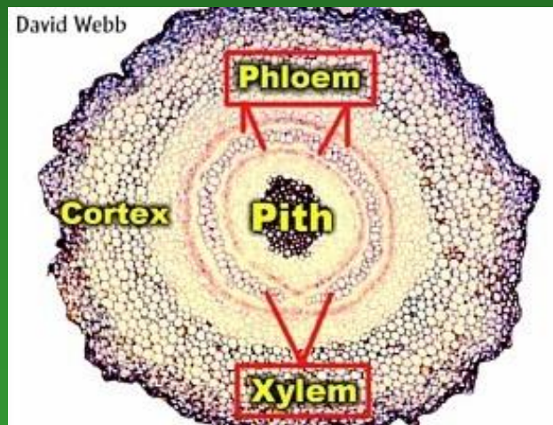
solenostélé
