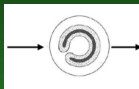
solenostélé
