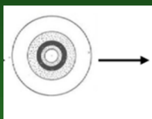
sifonostélé
