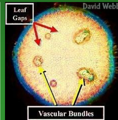
diktyostélé
