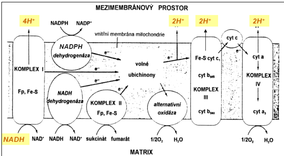
Hlavní proteinové komplexy ve vnitřní membráně mitochondrie a jejich součinnost při přenosu elektronů
