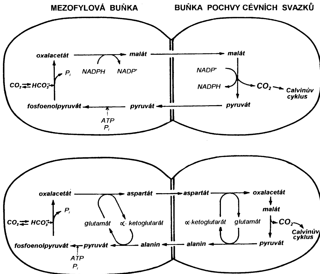
Schema dvou variant fixační cesty C 4 : varianta s transportem malátu (nahore) a s transportem aspartátu (dolní část obrázku). Existují i další modifikace C 4 -metabolismu.
