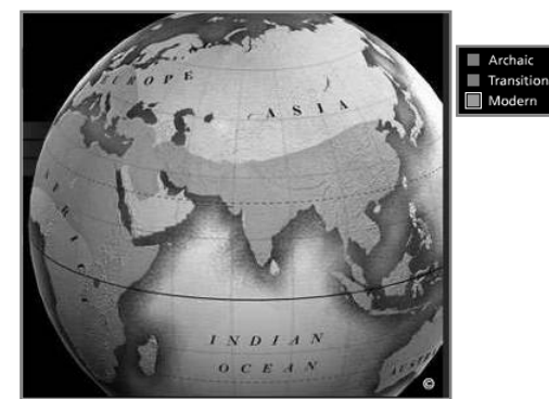
Multiregionální model
