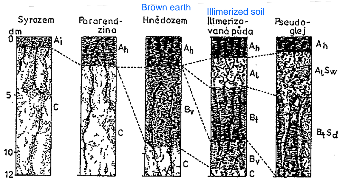
Vývoj půdy na písku (nahore) a spraši (dole) podle Mückenhausena (1975)
