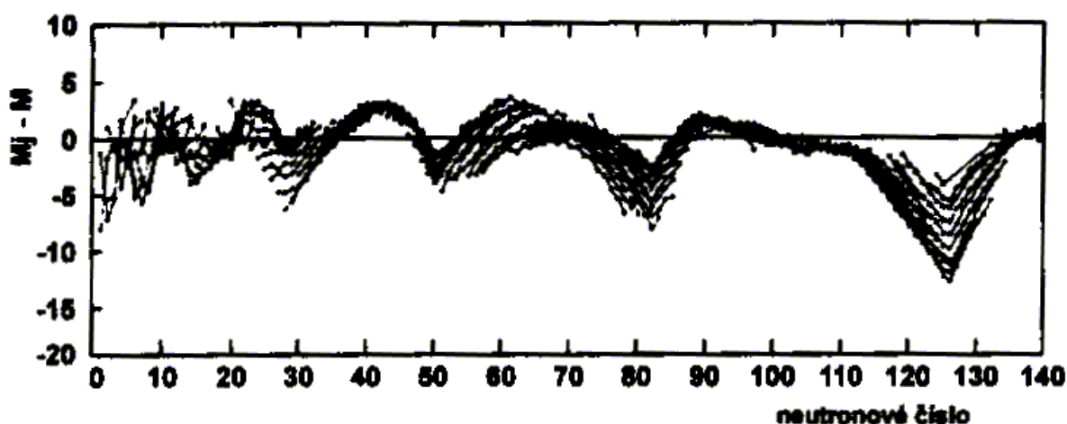
Obrázek 6: Rozdíl skutečných a vypočtených hmotností jader v závislosti na neutronovém čísle (čarami jsou spojeny izotopy). Stabilizaci jader je zřetelně vidět v oblasti N = 28, 50, 80 a 126 . Převzato z [38].
