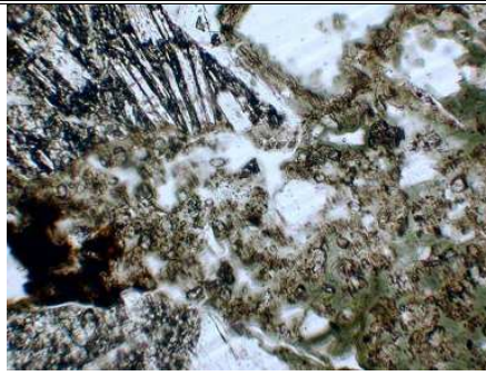
hyalinní –mikrostruktura PPL
