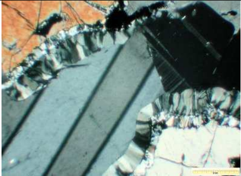
kelyfické lemy kolem olivínu jsou tvořené dvěma zónami jehličkovitého amfibolu, které vznikají všude, kde se stýká olivín s plagioklasy.
