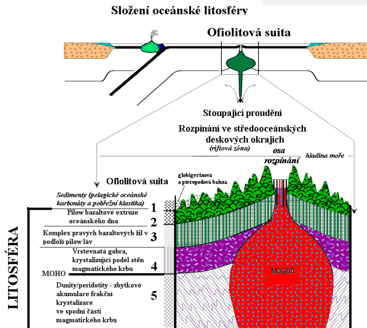
Obr. 28 Rozpínání oceánského dna tvorba MORB bazaltů
