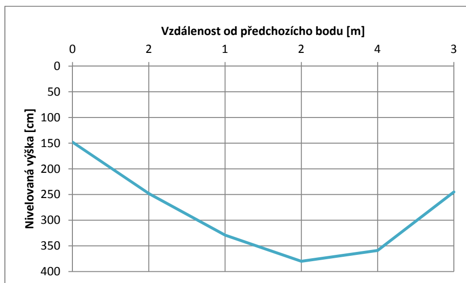
Obr. 3: Příčný profil koryta 3
