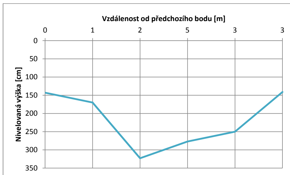
Obr. 2: Příčný profil koryta 2
