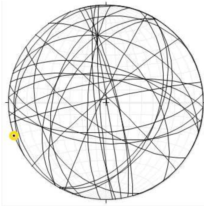
Obr. 2: Obloukový model druhého měření
