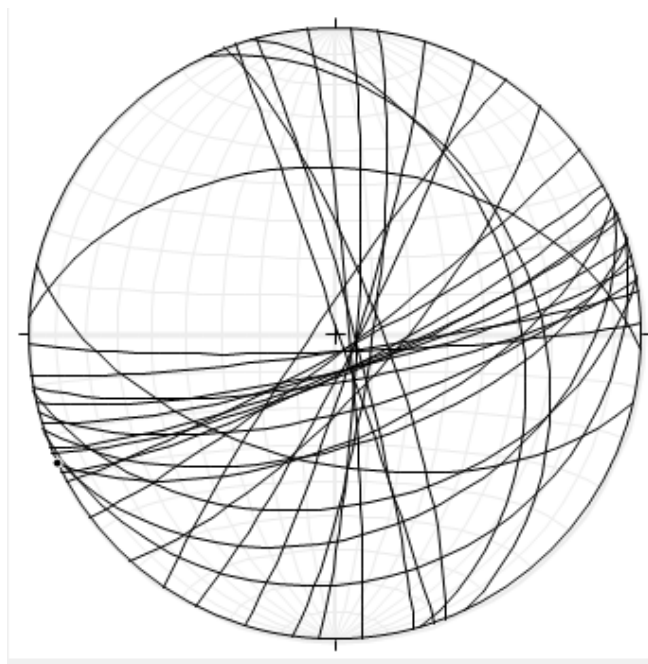
Obr. 1: Obloukový model prvního měření
