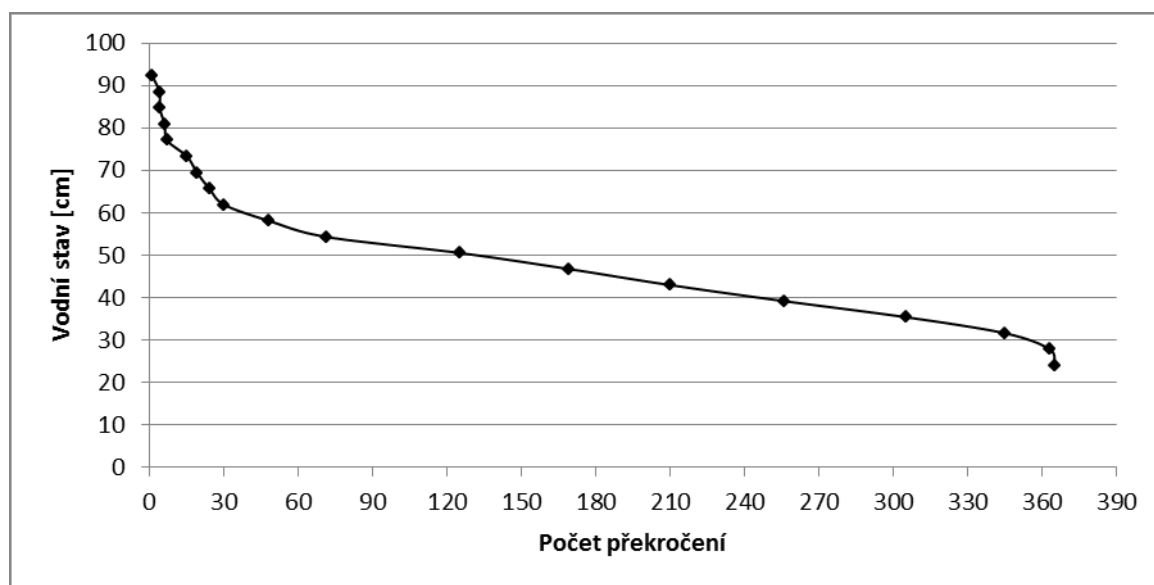
Obr. 2 Čára překročení denních vodních stavů na řece XY na stanici XY v hydrologickém roce XZ (zdroj dat: IS, studijní materiály, 2015)
