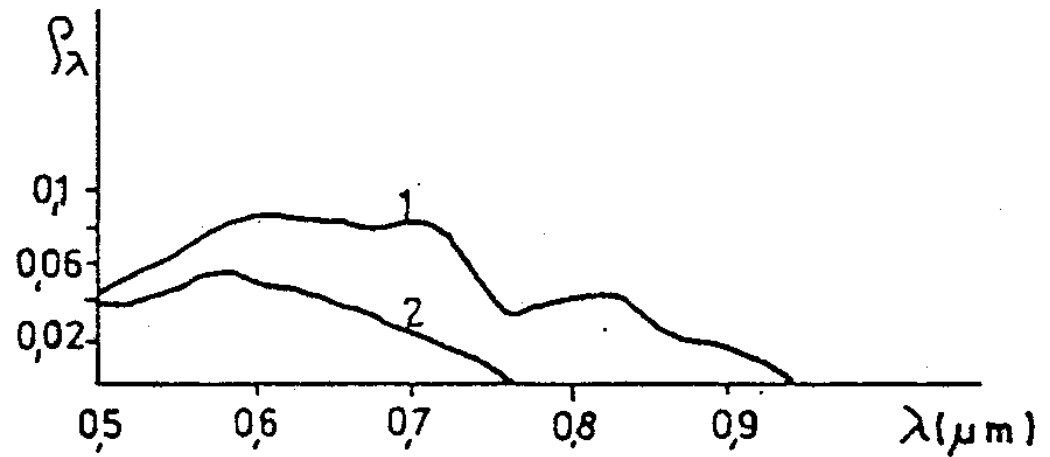
Spektrální odrazivost vody s vysokým obsahem kalu (1) a čisté jezerní vody (2)
