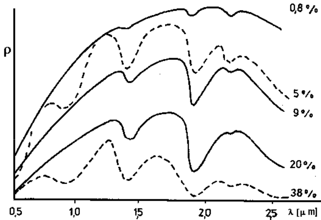
Schematizované spektrální chování různě vlhké prachovité hlíny (plná čára) a jílu (čárkovaná čára) v části viditelného a blízkého infračerveného elektromagnetického spektra
