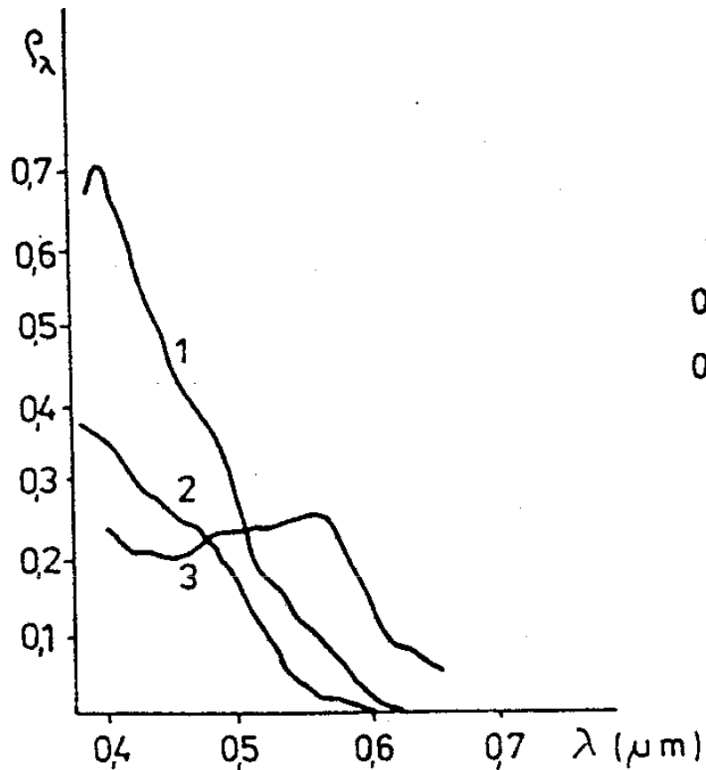
Spektrální odrazivost mořské vody s různým obsahem chlorofylu: 1 – velmi nízký obsah, 2 – nízký obsah, 3 – vysoký obsah
