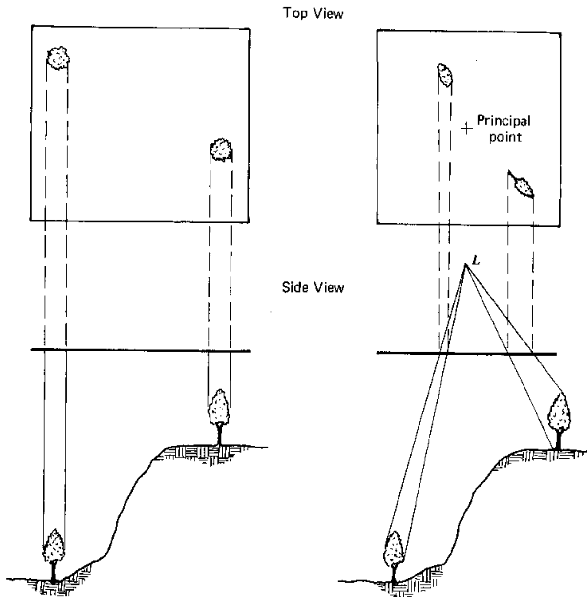
Rozdíly v geometrii mapy (ortogonální projekce) a letecké fotografie (centrální projekce)
