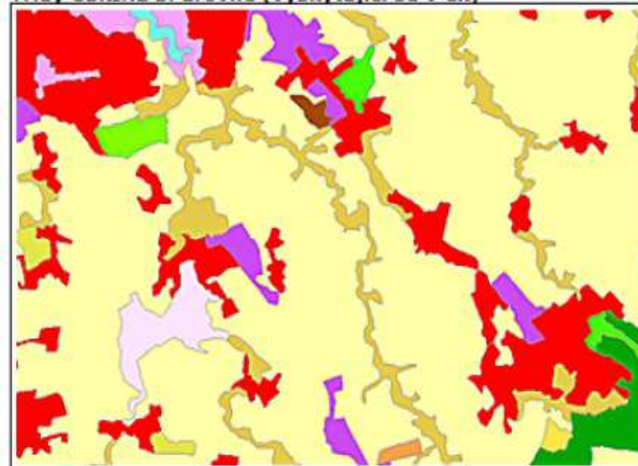
Třídy CORINE 3. úrovně (vyskytující se v ČR)
