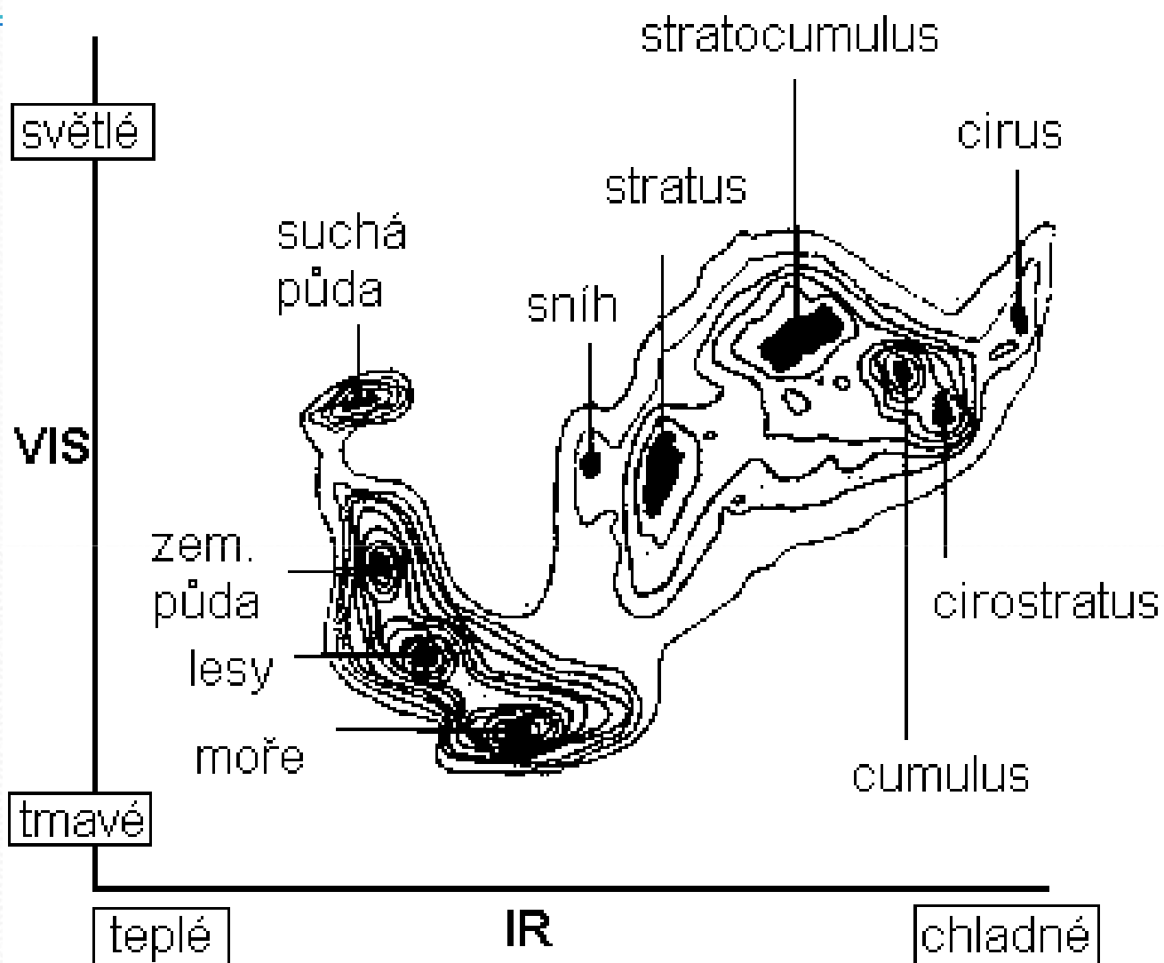
Interpretace druhů povrchů na základě korelačního pole DN hodnot viditelného (VIS) a infračerveného (IR) pásma
