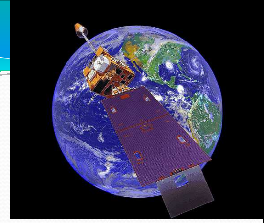
FY-2 GMS-5
