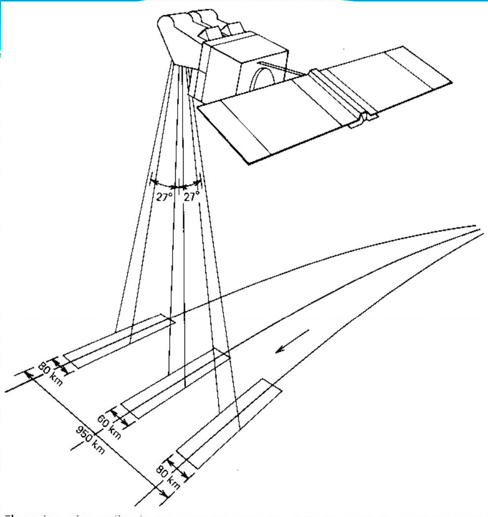
Princip vytváření digitálního modelu terénu z dvojic obrazových záznamů družice SPOT
