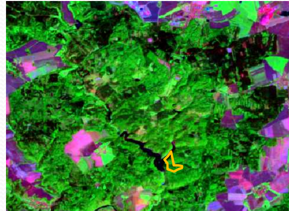
Syntéza v nepravých barvách (7,4,2)
