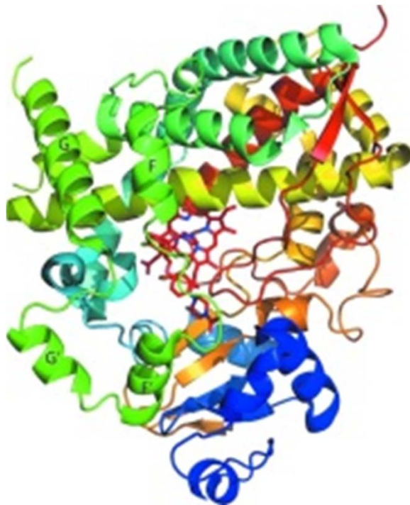
CYP3A4 s navázaným inhibitorem
