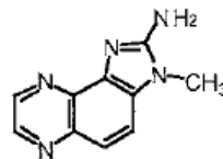
IQx
