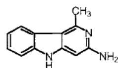
Trp-P-2
