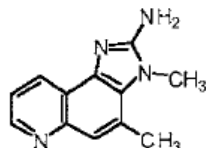
MeIQ
