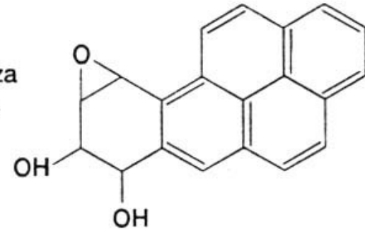
9,10-epoxy-benzo[a]pyren-7,8-diol
