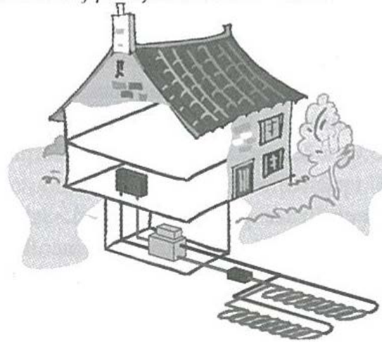
Obr. 8 Primární zdroj pro systém země – voda.
