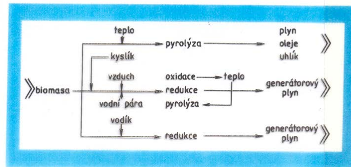
Procesy zplyňování
