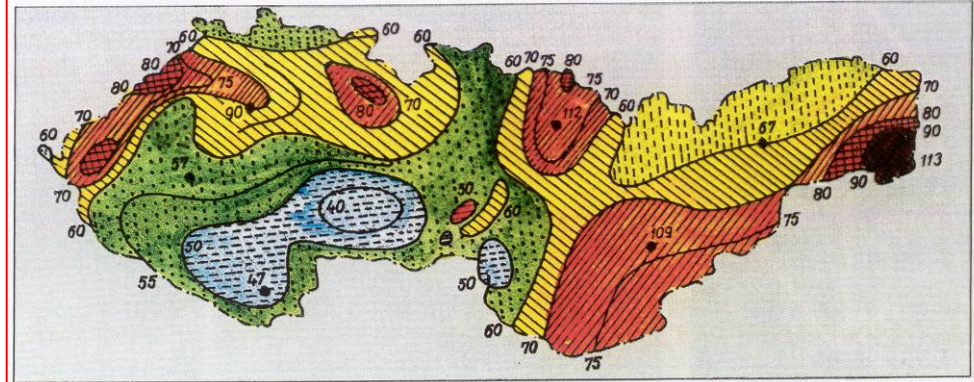
Tepelný výkon geotermálních zdrojů na území ČSFR. Isočary vymezují místa shodné geotermální aktivity (mW/m²).
