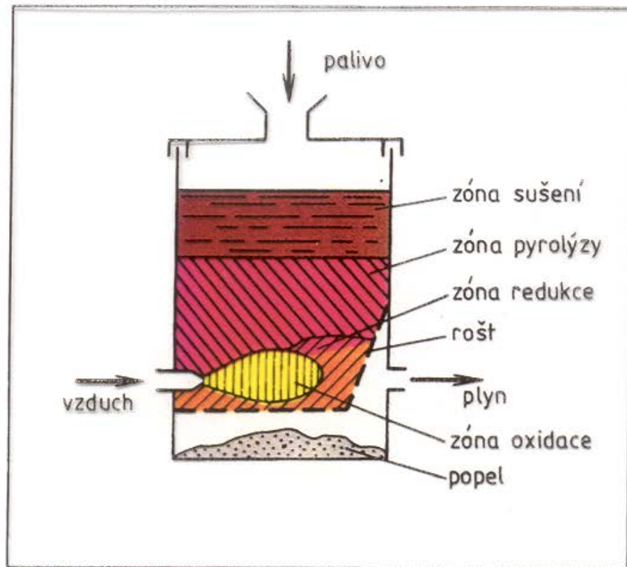
Zplyňovač s příčným prouděním
