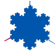
KLASICKÁ KOCHOVA VLOČKA (PO 4. KROU ALEDRITMU)
