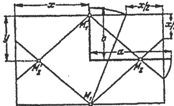
DVAŘ NA CHRÁMOVÉ STĚNĚ (LUXOR, -12. STOLETÍ) A JEHO KONSTRUKCE ↗
