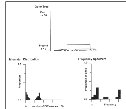
Model s konstantní velikostí
