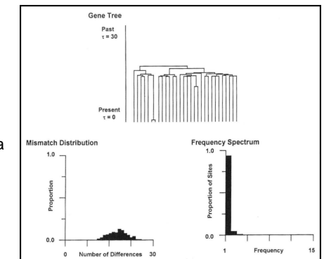
Model s populační explozí
