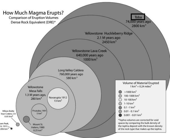
Srovnání velikosti výbuchu supersopky Toba s ostatními supervulkány.
