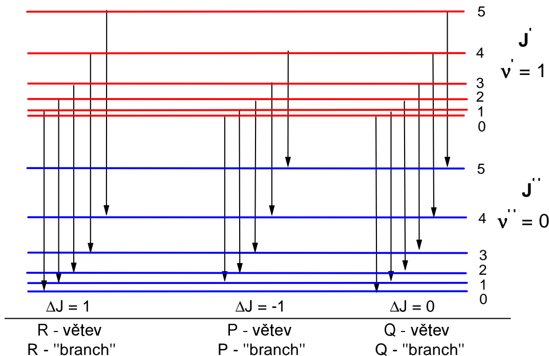
Figure 3: Princip vzniku rotačních R, P a Q větví pro případ, kdy J=N .
