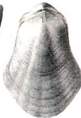
Pentamerida
