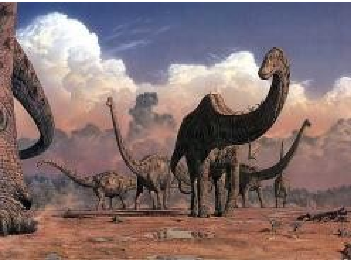
„ Seismosaurus “
