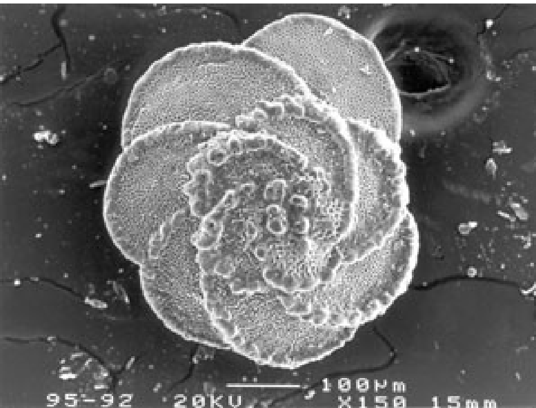
Globotruncana sp., Foraminifera, sv. křída, Alicante, Španělsko
