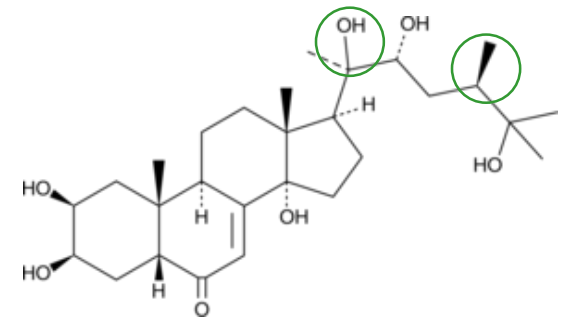
makisteron A
