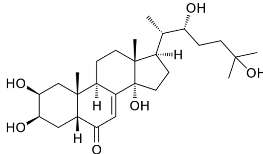
ekdyson
