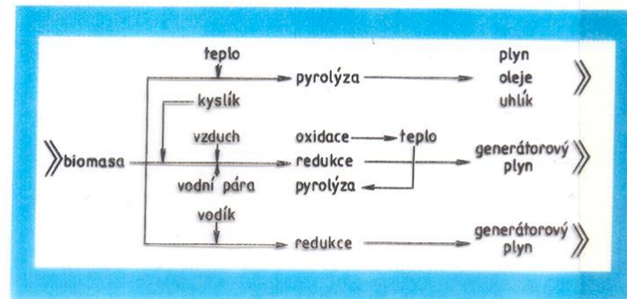
Procesy zplyňování
