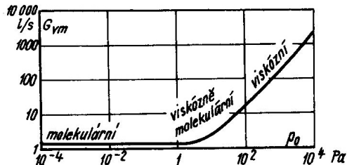
Obr. 2.39. Vodivost potrubí G jako funkce tlaku p_0 v širokém oboru tlaků. Vzduch o teplotě 20^\circ\text{C} , potrubí o L = 10\text{ cm} a D = 1\text{ cm}
