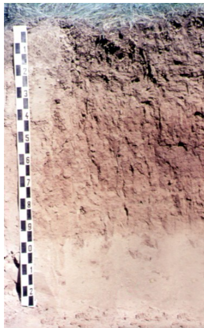
Obr. 2 Půdní profil subtypu HNm hnědozem modální na vybraném území. Zdroj: TKSP ČR, [www]
