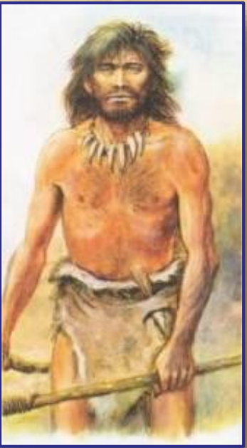
Homo sapiens
