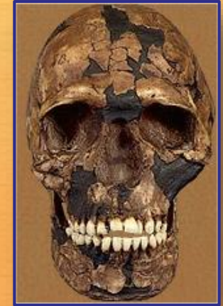
Homo sapiens
