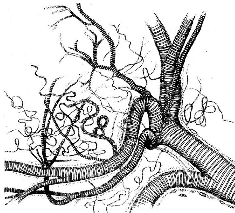
Tracheje - vzdušnice
