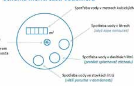
Schéma měřící části vodoměru
