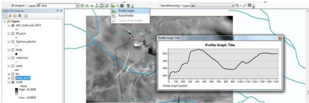
Obr. 18 Výškový profil
