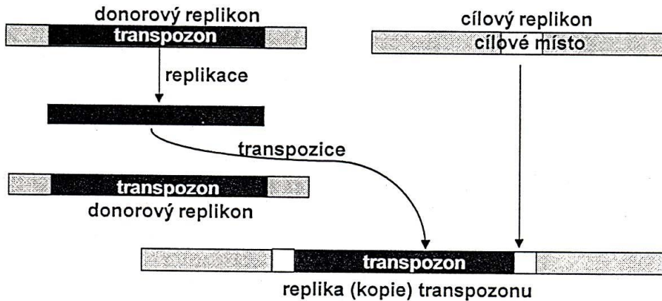
Obr. 404 Replikativní transpozice
