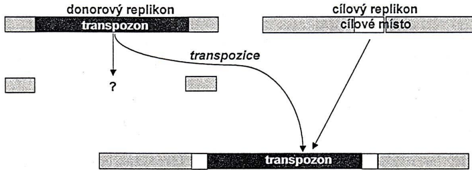
Obr. 403 Konzervativní transpozice
