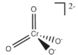
\text{CrO}_4^{2-} chromate anion
