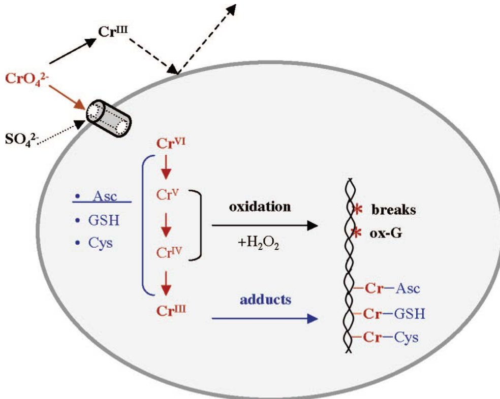
\text{SO}_4^{2-} sulfate anion
