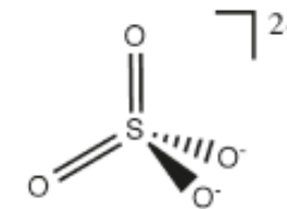
\text{SO}_4^{2-} sulfate anion
