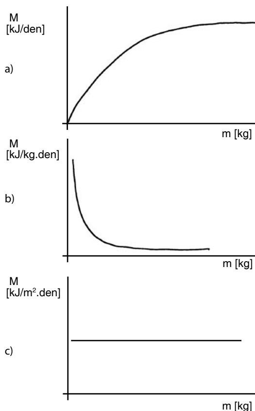
Obr. 5.8. Vztahy mezi metabolizmem (M) a tělesnými parametry. a) absolutní hodnota M (energetických toků) roste s velikostí těla, b) vzhledem k jednotce hmotnosti těla (jedné buňce) M směrem k větším živočichům klesá, c) na jednotku tělesného povrchu je M stejný bez ohledu na hmotnost – M je těsně vázán na povrch.
