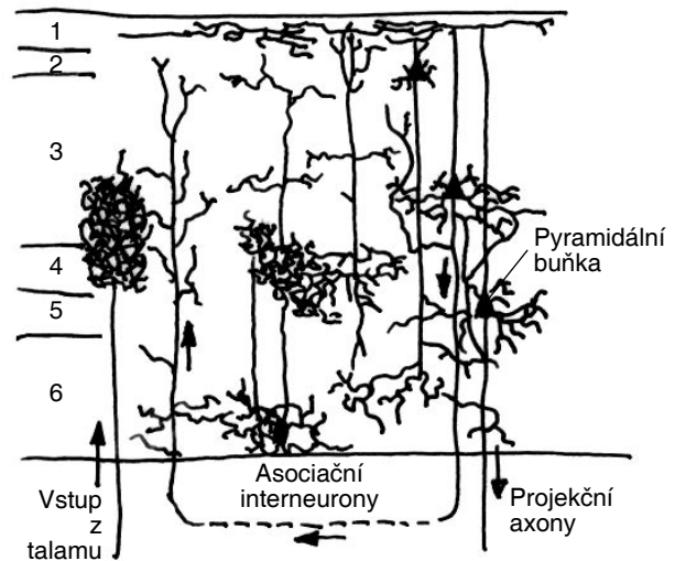
Obr. 16.11. Šest vrstev horizontálního členění kůry savců. Do sloupce – modulu – vstupuje aferentní informace z talamu, po zpracování asocičními interneurony eferentní motorický výstup odchází opět do spodních vrstev.
