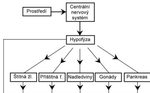
Obr. 18.3. Regulace nervovým systémem je nadřazena nad autoregulaci biorytmů.
