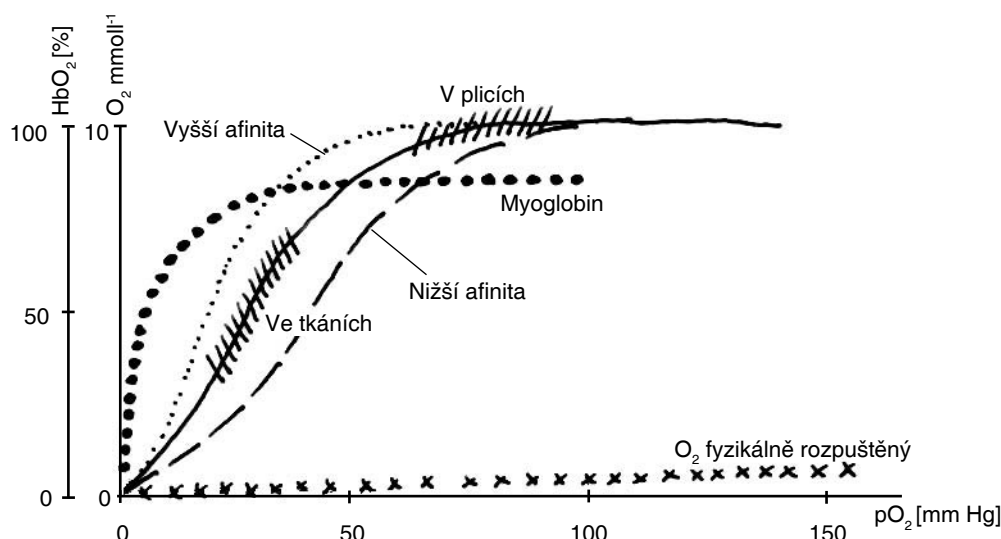
Obr. 12.6. Saturační, vazebné křivky hemoglobinu (Hb) mají sigmoidní tvar. Afinita Hb ke kyslíku se může měnit (vliv teploty, pH), posun křivky doprava znamená nižší afinitu. Šrafovaně jsou pracovní rozsahy: ve tkáních je nižší pO_2 a křivka je nejstrmější – O_2 se nejlépe uvolňuje. V plicích je křivka plochá – důsledky změn pO_2 (např. s nadmořskou výškou) jsou malé. Myoglobin má jen jednu jednotku a jiný tvar křivky.
