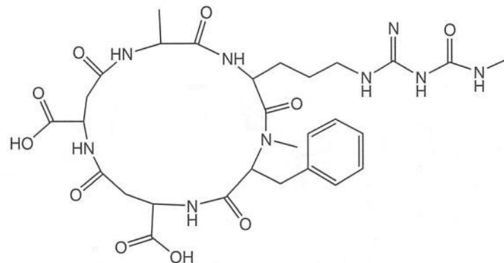
Argifin
