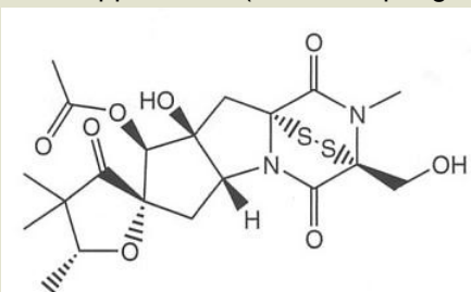
Sirodesmin PL
