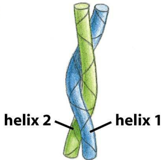
(B) HELIX-HELIX
