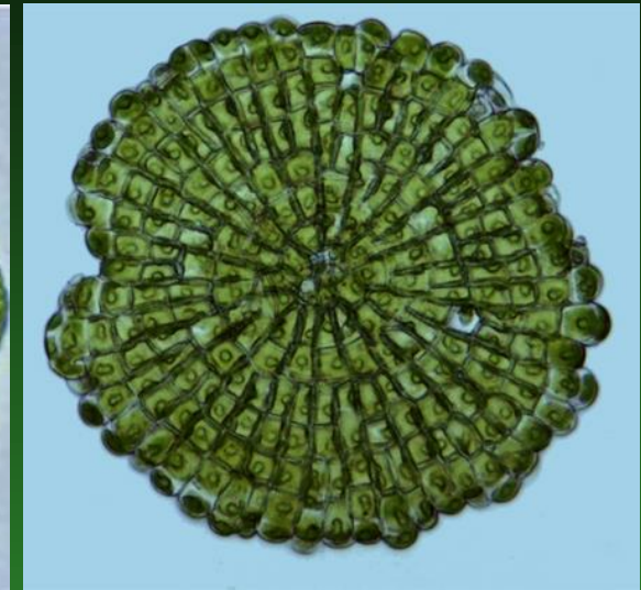
Coleochaete
