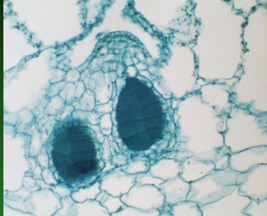
zanořená antheridia
