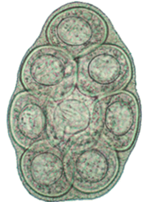
Dipylidium caninum
