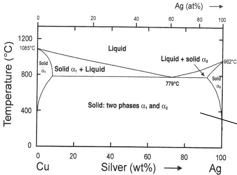
Rovnovážný fázový diagram Cu-Ag
