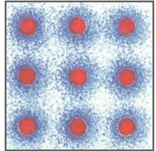
Elektronový mrak – kovová vazba
