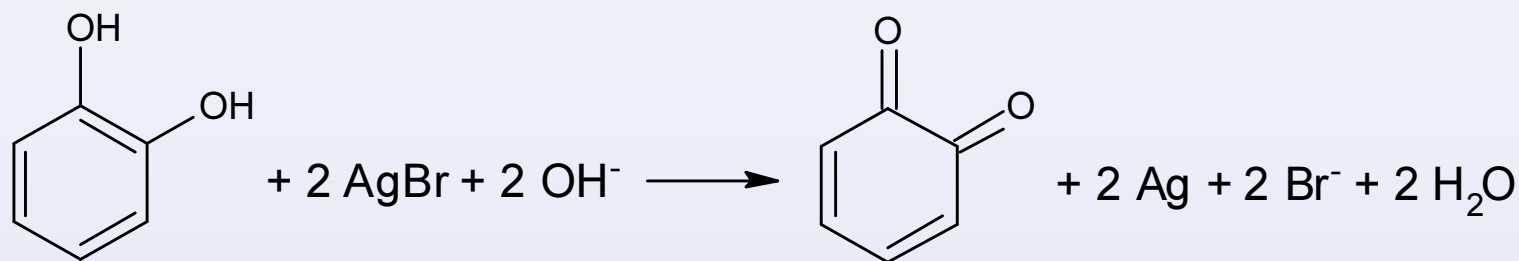
1,2-benzendiol (pyrokatechol)
