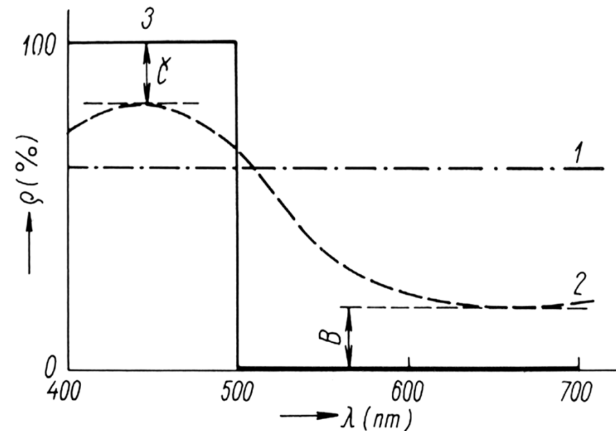
Spektrální reflektance ideálních a skutečných povrchových barev
