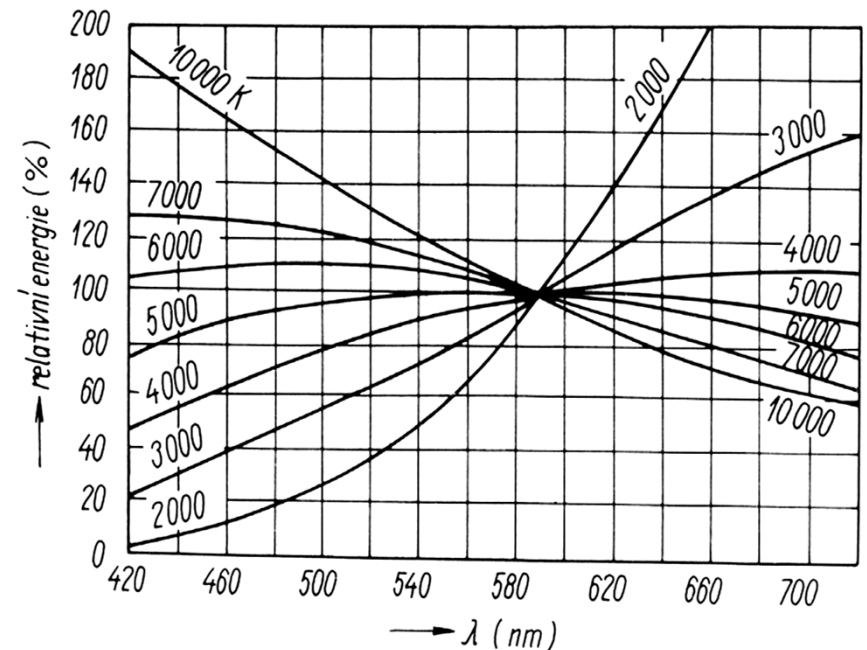
Rozložení energie ve spektru absolutně černého tělesa
