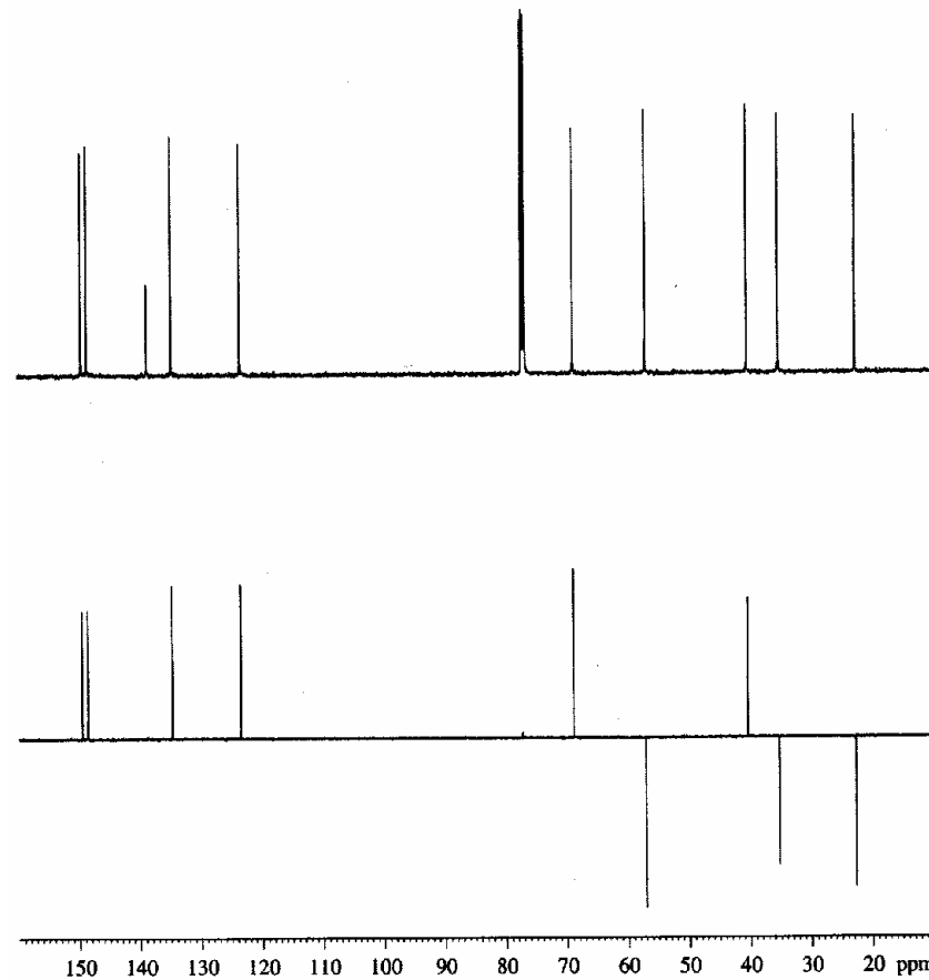
13 C NMR
