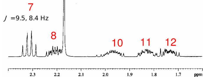
1 H NMR
