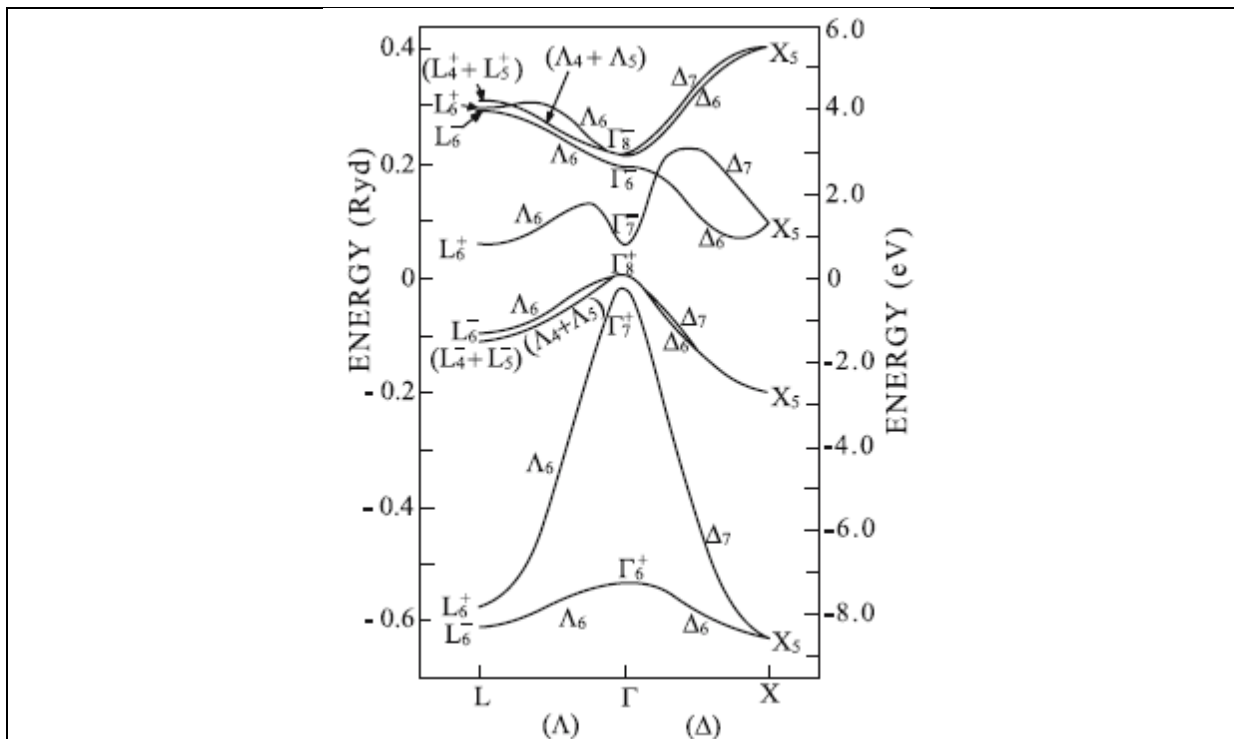
Pásová struktura Ge se započtením SO interakce (Dresselhaus). Pozor na valenční stavy s nejmenší energií.
