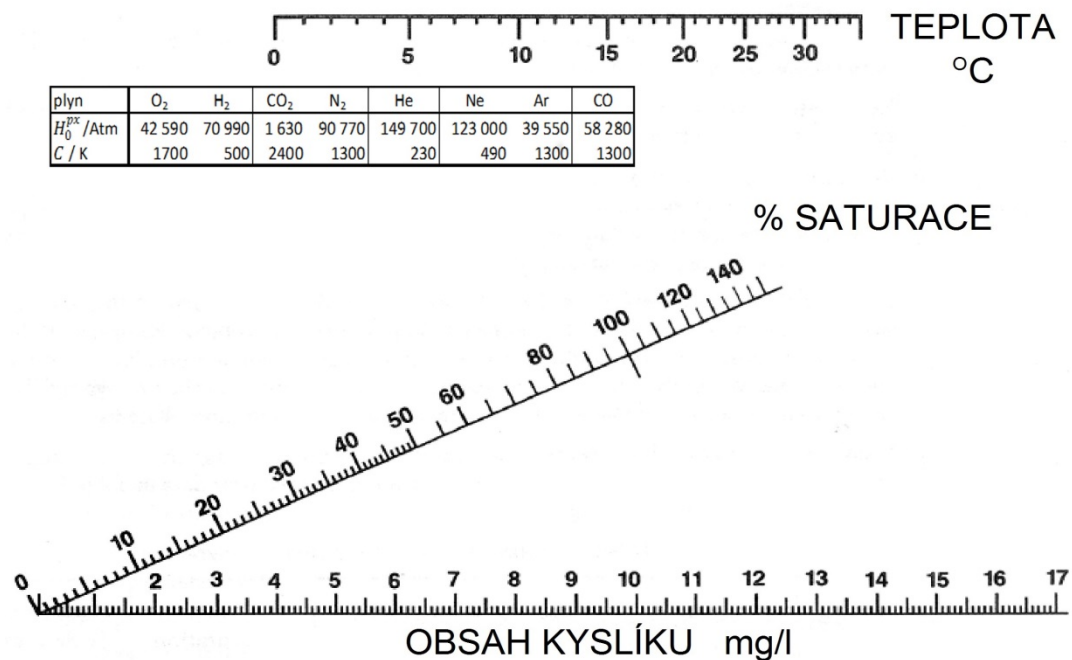
OBRÁZEK 1: Monogram teplotní závislosti rozpustnosti kyslíku ve standardní atmosféře při různém stupni saturace vody. Vložená tabulka uvádí parametry H_0^{px} a C teplotní závislosti Henryho konstanty H^{px} různých plynů rozpouštěných v čisté vodě.
