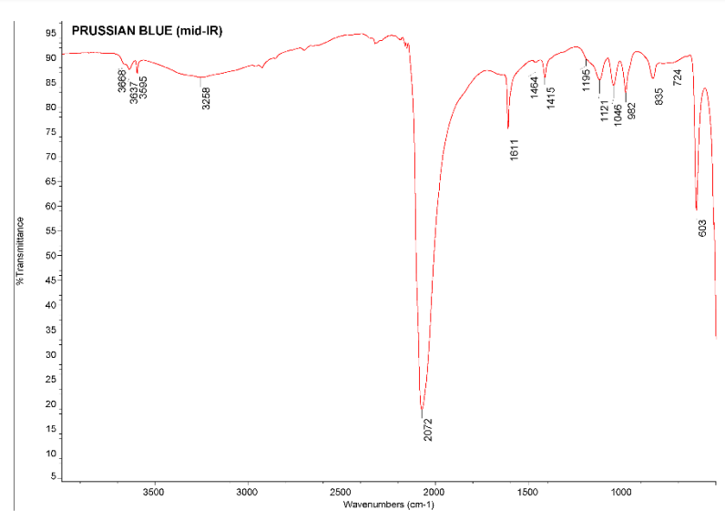
Fig. 21 IČ spektrum
