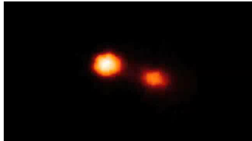
\beta Lyrae
