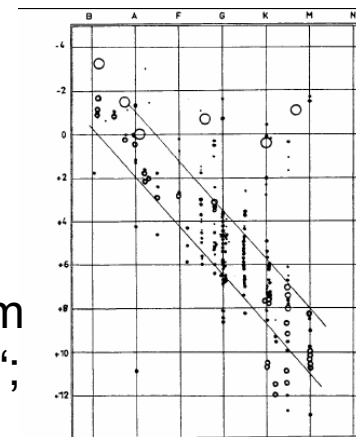
RUSSELL's erstes Diagramm (veröffentlicht in Popular Astronomy, 1914) Abzisse: Spektraltyp. System MITT CANNON. Ordinate: Absolute Helligkeit. ○ • Sterne mit einem Fehler der Parallaxe < 42% ○ • Sterne mit einem Fehler der Parallaxe > 42%
